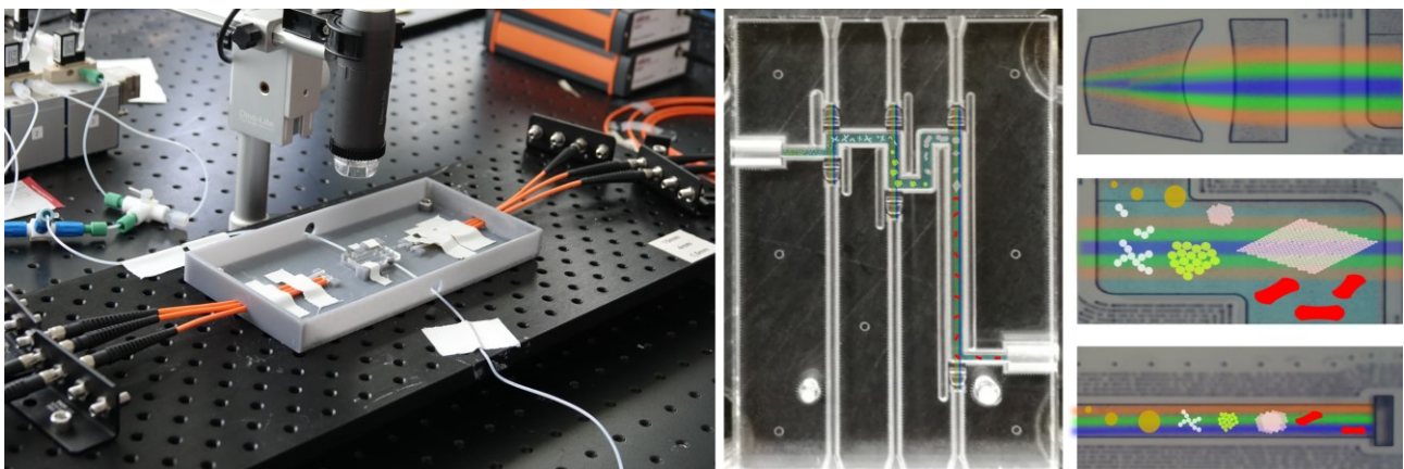
Figure 1 Photographies d'une puce microfluidique pour la caractérisation de nano- et micro-suspensions par extinction UV-NIR [5]
